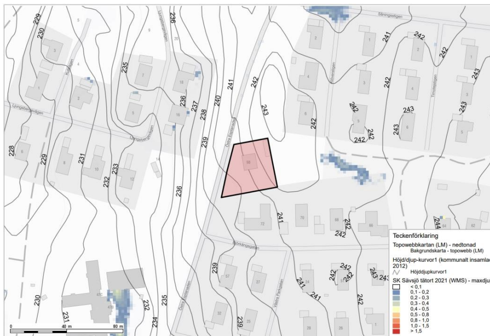
Figur 5: Karta med höjdkurvor och maxdjup från översvämningsskartering Sävsjö (2021)
